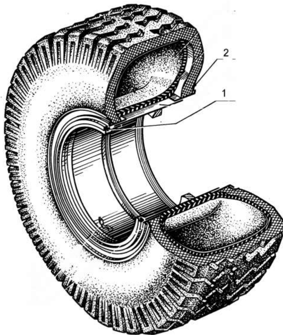
Рисунок 7 – Колесо с шиной (086CX 12,8-06.020)
